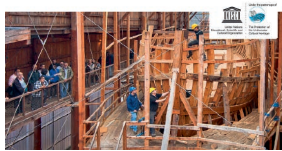
Construcción de la nao San Juan en Albaola.
